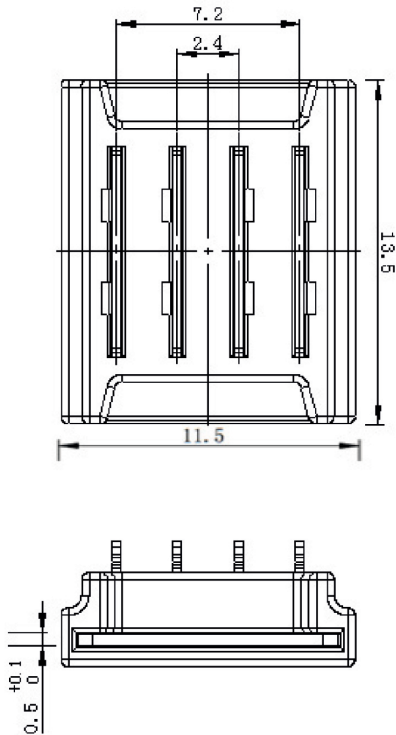
SMD 10mm 灯带 - 灯带 4 芯连接器 HR-S-SMD-4PIN-10MM-A
