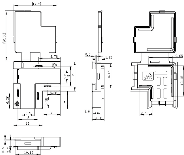
COB 10mm 灯带 - 灯带 2 芯 T 型连接器 HR-S-SC-2PIN-10MM-T
