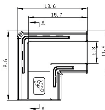
COB 10mm 灯带 - 灯带 2 芯转角连接器 HR-S-SC-2PIN-10MM-L
