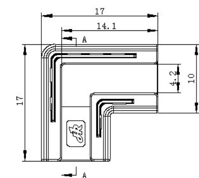
COB 8mm 灯带 - 灯带 2 芯转角连接器 HR-S-SC-2PIN-8MM-L
