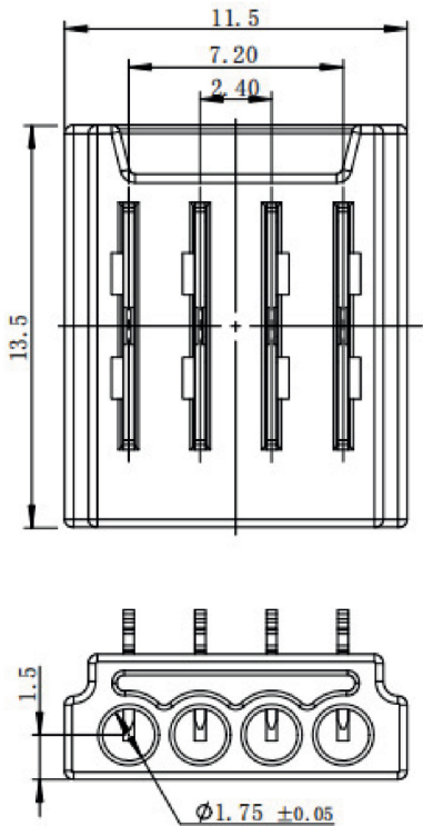
SMD 10mm 灯带 - 线 4 芯连接器 HR-S-SMD-4PIN-10MM-D HR-S-SMD-4PIN-10MM-B HR-S-SMD-4PIN-10MM-C
